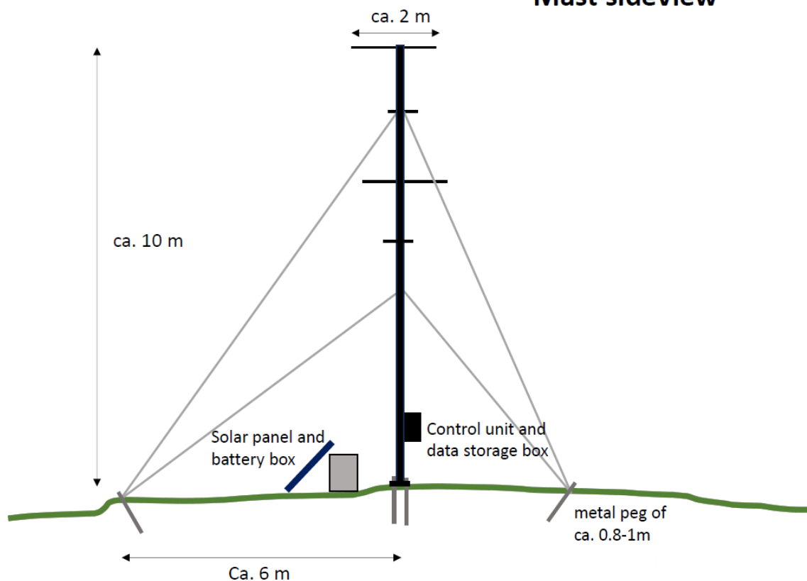
Principskitse over mast. Modtaget med ansøgningsmaterialet.
