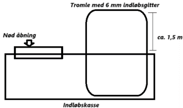
Figur 2: Indløb med tromle og nødåbning
