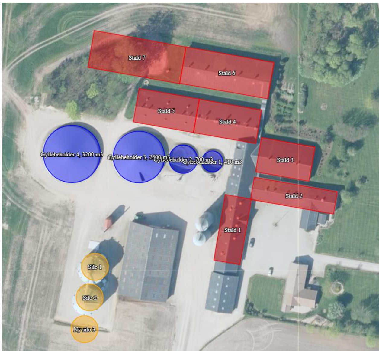
Figur 1. Oversigt over staldafsnittenes placering samt placering af den nye silo
