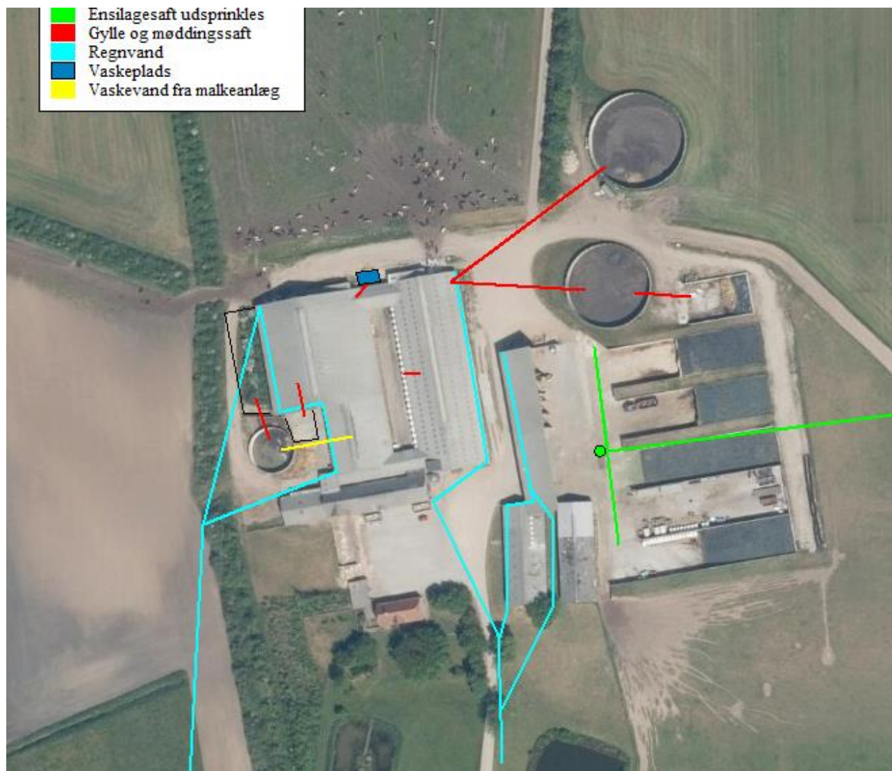
Figur 3. Afløbsplan
