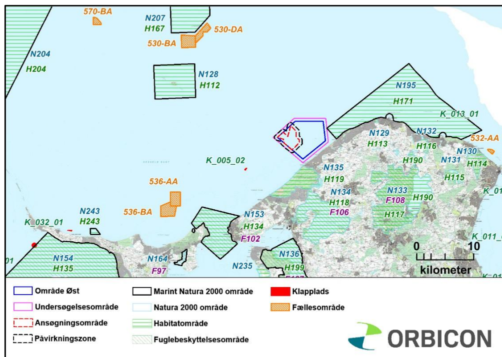
Figur 3-2. Oversigt over omkringliggende råstofindvindingsområder (fællesområder), klappladser og Natura 2000-områder i forhold til Område Øst.
