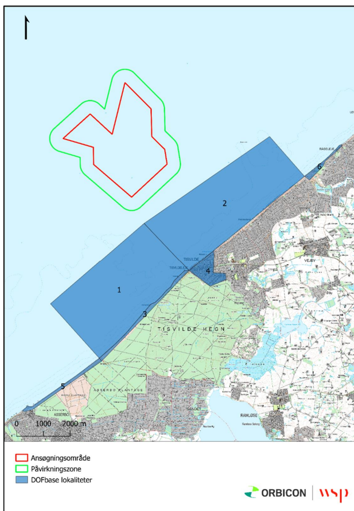
Figur 8-16. Anvendte kystnære samt marine DOF-base lokaliteter nær område Øst. Lokalitetsnumre: 1) Havet ud for Tisvilde hegn, 2) Kattegat ml. Rågeleje og Tisvildeleje, 3) Tisvildekysten, 4) Tisvildeleje, 5) Asserbo strand (Melby strand) og 6) Rågeleje strand. Indtil 2018 omfattede lokaliteterne 3-6 på dette kort observationer af havfugle set fra land.
