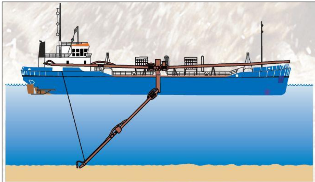
Figur 3-3. Skitse af metoden bag slæbesugning (Kystdirektoratet, 2012).
