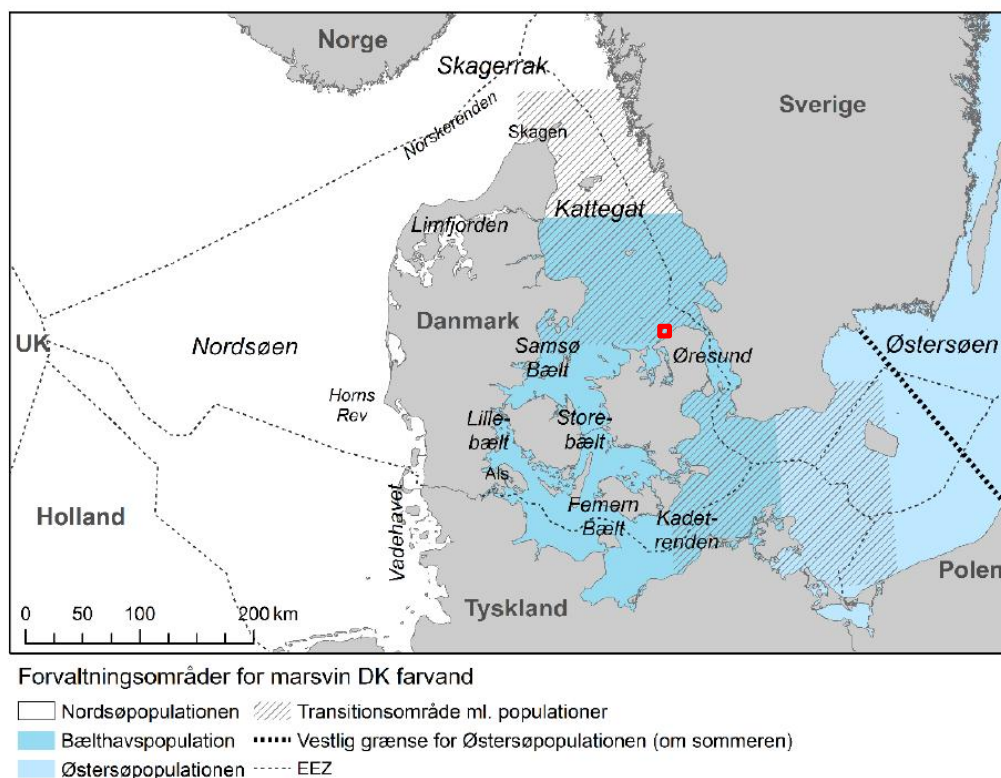
Figur 8-19. Kort over forvaltningsområderne for de 3 populationer af marsvin i danske farvande og i vores nabolande. Stiplede linjer viser nationalgrænserne (EEZ). Skraverede områder indikerer transitionsområder mellem de tre populationer. Ansøgningsområdets ca. placering er angivet med rød firkant på figuren. Kilde: (Sveggard et al., 2018).
