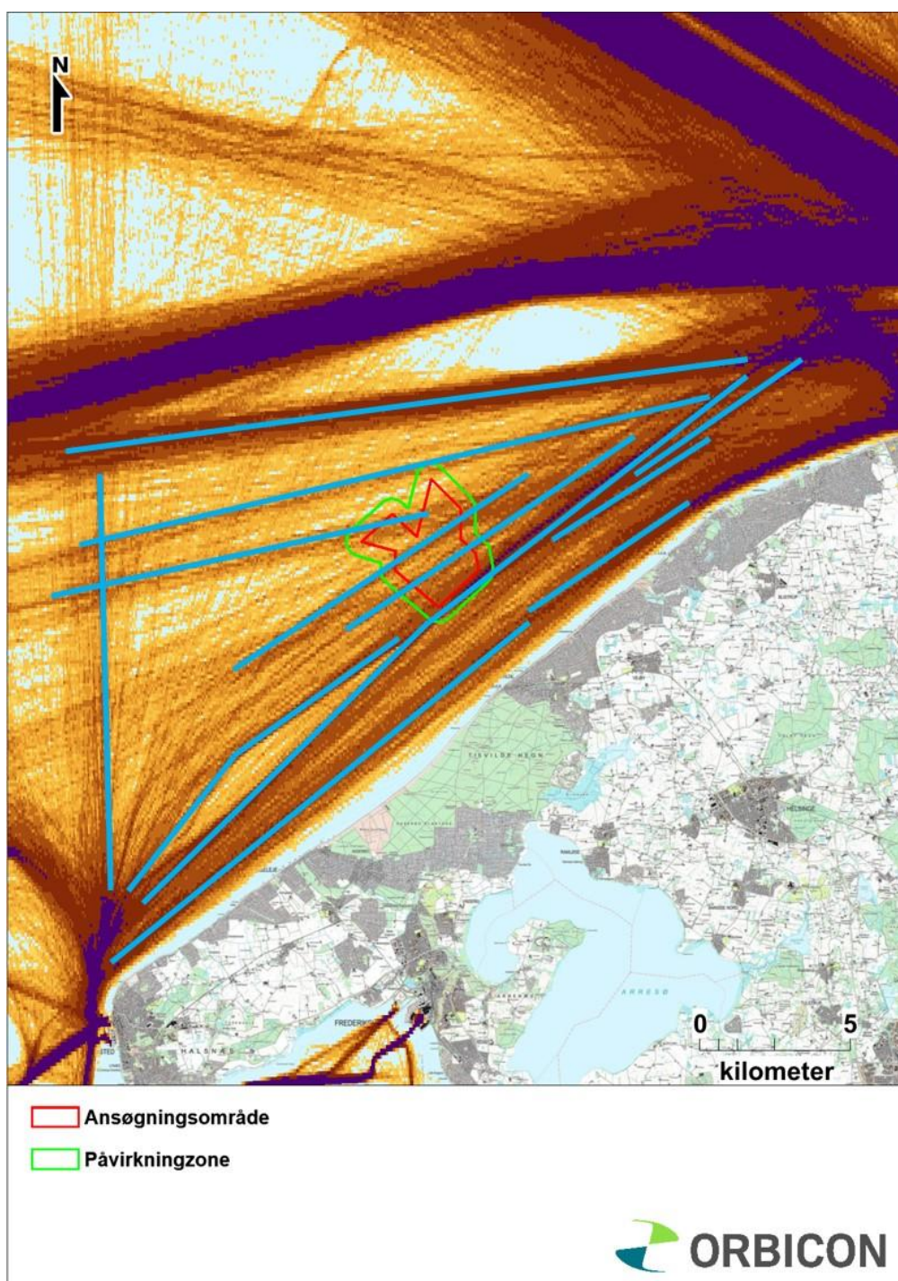
Figur 8-31. Dominerende sejlruiter i området omkring ansøgningsområdet.
