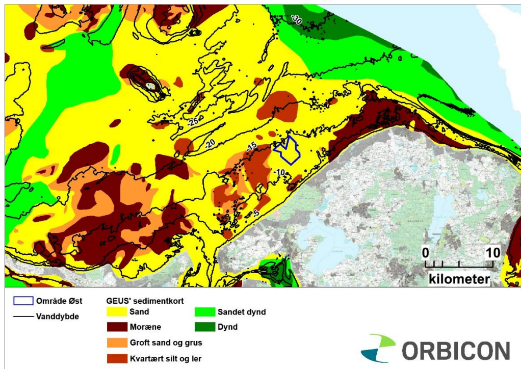
Figur 8-3. Fordelingen af overfladesedimenter i det sydlige Kattegat (GEUS, 2019b). På kortet er angivet beliggenheden af ansøgningsområdet for Område Øst.
