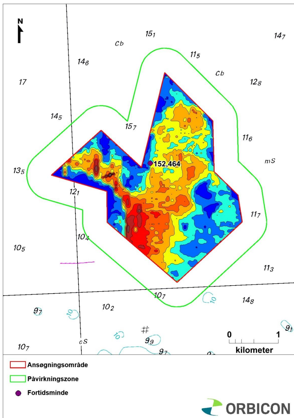
Figur 8-28. Kort over registrerede fund og fortidsminder inden for ansøgningsområdet. Som baggrund er angivet den kortlagte ressourcetykkelse inden for ansøgningsområdet. Den røde, gule og lyseblå farve indikerer henholdsvis en ressourcetykkelse på 3 til 3,5 m, 1,5 til 2 m og 1 til 1,5 m.
