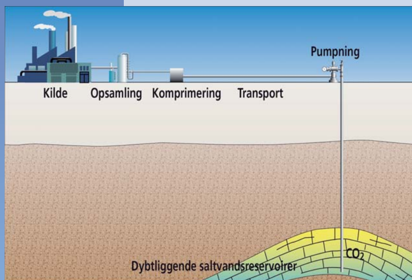
Figur 1 Stadier i geologisk lagring af CO 2 . Sikker og langsigtet lagring af CO 2 kræver en hel række processer som f.eks. opsamling, komprimering, transport og nedpumpning.
