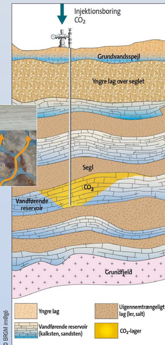
Figur 1 Den injicerede CO 2 , der er lettere end vand, stiger opad og stoppes af det overliggende og uigennemtrængelige segl.
