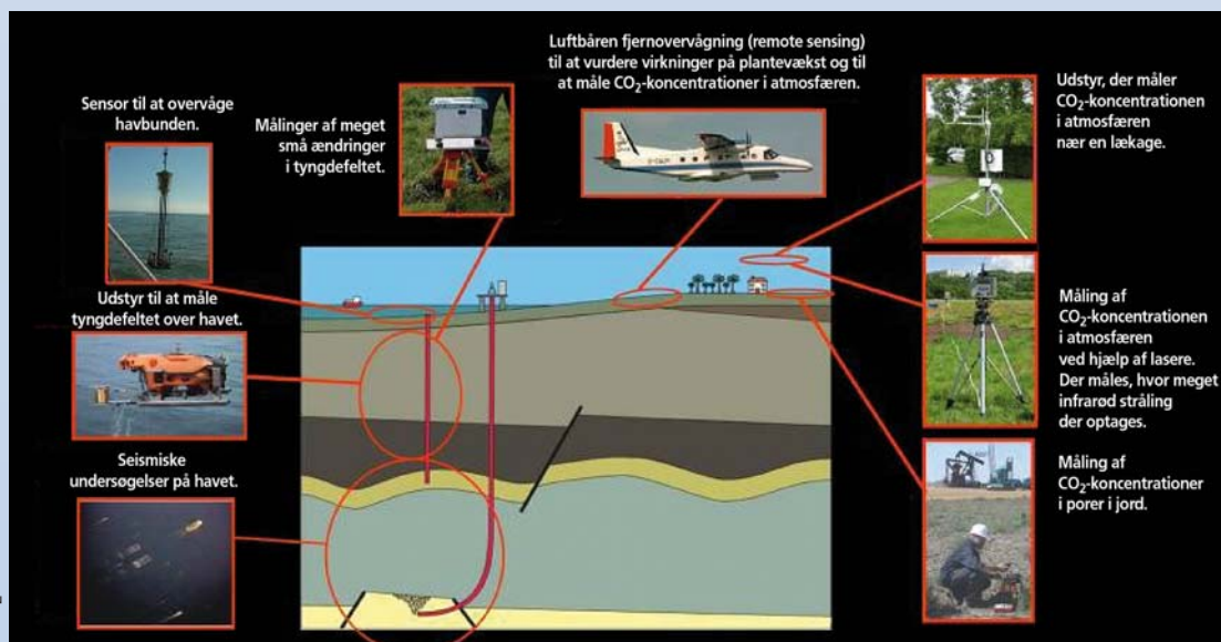
Figur 3 Et lille udvalg af de metoder, der kan bruges til at overvåge forskellige dele af et CO 2 -lager.
