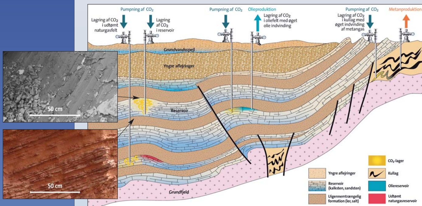
Figur 1 CO 2 pumpes ned i dybtliggende geologiske lag bestående af porøse og gennemtrængelige aflejringer (f.eks. sandsten som vises i det nederste indsatte foto), hvorover der ligger et uigennemtrængeligt lag (f.eks. lersten som vises i det øverste indsatte foto), der forhindrer CO 2 i at stige op til jordoverfladen. De primære lagringsmuligheder er: 1. Udtømte olie-/gasreservoirer med eventuel forøget udvinding af olie eller naturgas 2. Reservoirer med saltvand, der er uegnet som drikkevandsmagasin 3. Dybtliggende kullag, der lokalt kan anvendes til øget indvinding af metangas.
