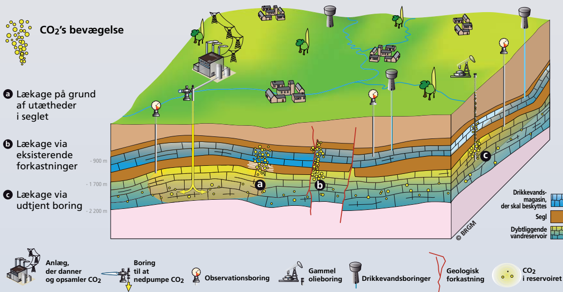
Figur 2 Eksempler på mulige lækager.
