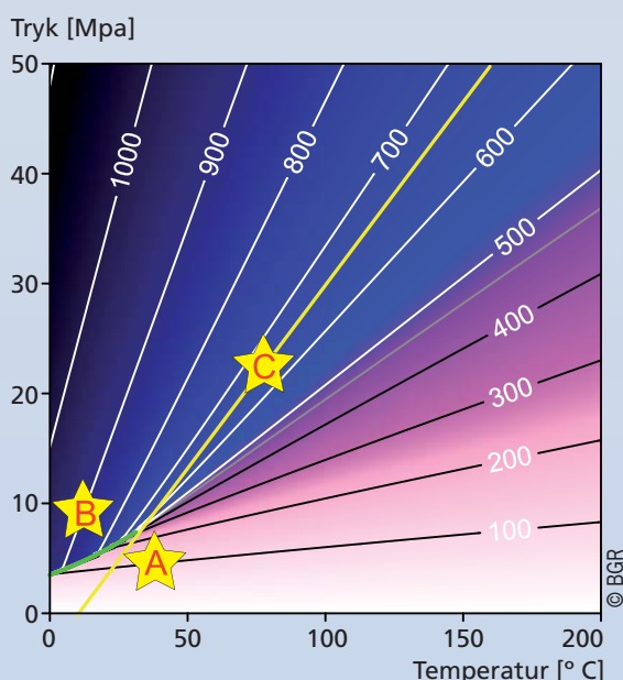
Figur 3 Tætheden af ren CO 2 (kg/m 3 ) i forhold til temperatur og tryk. Den gule linje angiver en typisk temperatur- og trykgradient i et sedimentbassin. Ved dybder på mere end 800 m (~8 MPa (Mega Pascal)) er forholdene i reservoiret med til at øge tætheden af CO 2 gassen (blå skygge). Den grønne kurve markerer CO 2 's overgang fra gas til væske fase. A, B og C angiver typiske tryk- og temperaturforhold ved henholdsvis opsamling, transport og lagring af CO 2 .
