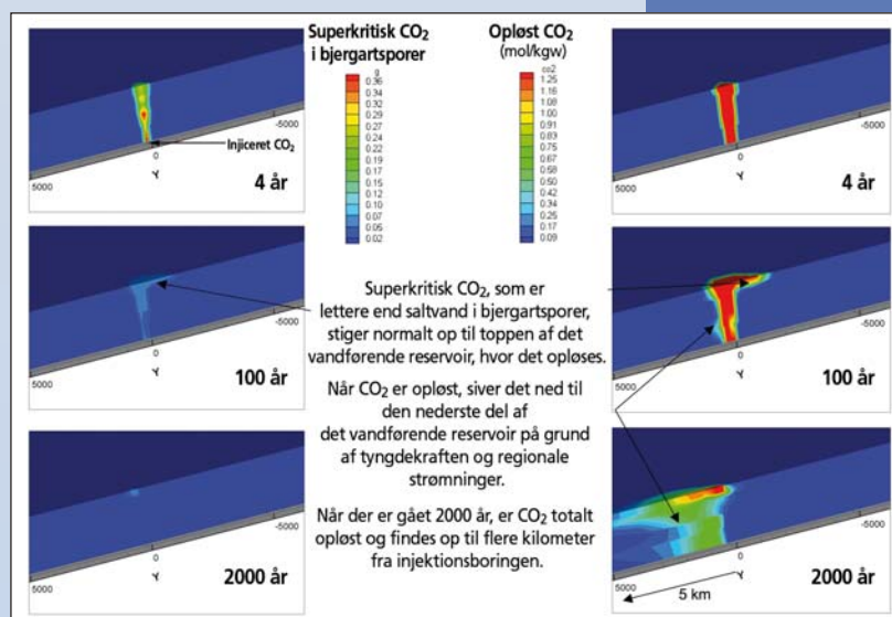
Figur 4 Tidimensional model, der viser, hvordan CO 2 har bevæget sig i et vandførende lag, når 150.000 tons er blevet injiceret i Dogger grundvandsreservoiret* i Frankrig over en periode på 4 år. Her vises superkritisk CO 2 (til venstre) og CO 2 opløst i saltvand (til højre) henholdsvis 4, 100 og 2000 år efter, at nedpumpningen begyndte. Simuleringerne er baseret på data fra undergrunden og fra forsøg.
