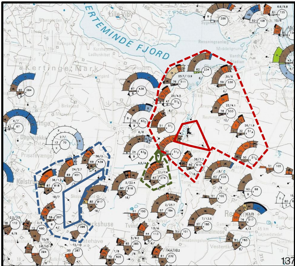
Fig. 18. Udsnit af geologisk basisdatakort 1313 i Kerteminde (Fra Jakobsen, 1993). Signaturforklaring: se fig. 7. Indvindingsboringerne til Kerteminde Vandværk er afgrænset til tre områder. Rød stregsignatur viser tætliggende borer i nordligt område. Grøn signatur viser en boring i mellemliggende område og blå signatur viser borer i sydligt område. De punkterede linjer viser de tilhørende cirkeldiagrammer (Fra Ernstsens et al., 2012).
