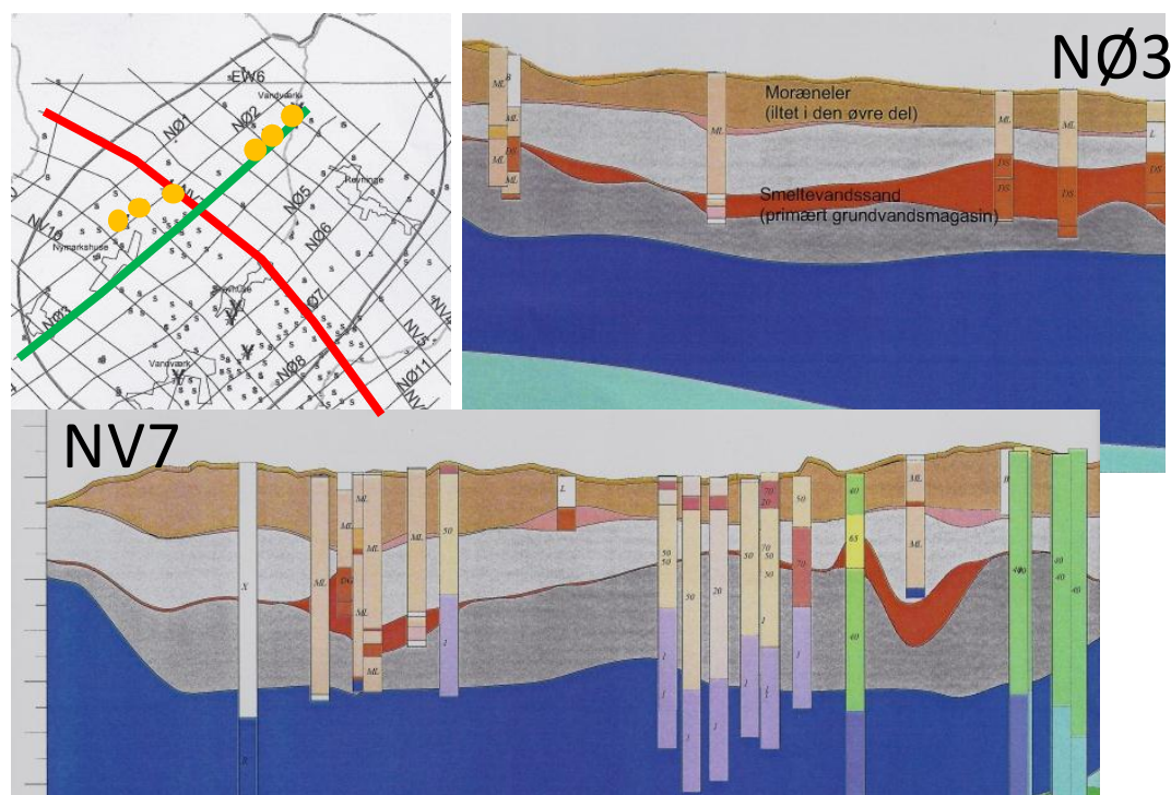
Fig. 17. To tolkede profiler fra indsatsområde Kerteminde udført af Hedeselskabet (2004). De to profilinjer ses på kortet, hvor profil NØ3 ses som en grøn linje og NV7 som en rød linje, mens de gule prikker er borer. Signaturer: Brun: moræneler; Grå: sandet moræneler; Mørkegrå: kompakt moræneler; Rød: smeltevandssand; Blå: palæocæn Kerteminde Mergel; Grøn: palæocæn Grønsandskalk (fra Ernstsens et al., 2012).
