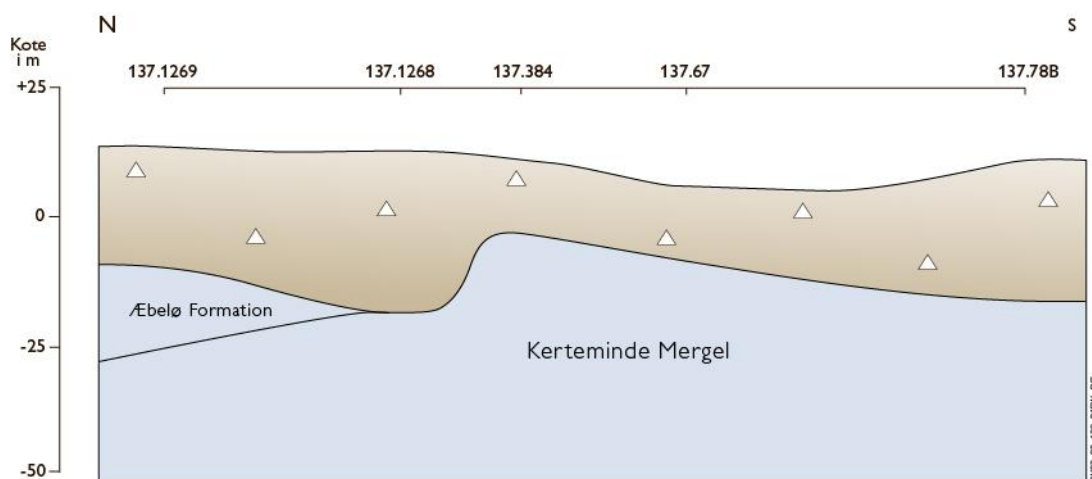
Fig. 9. Profil nord-syd gennem området fra Kertinge til Tværgyden. Profillængde 4,2 km. Overhøjning ca. 20 X.
