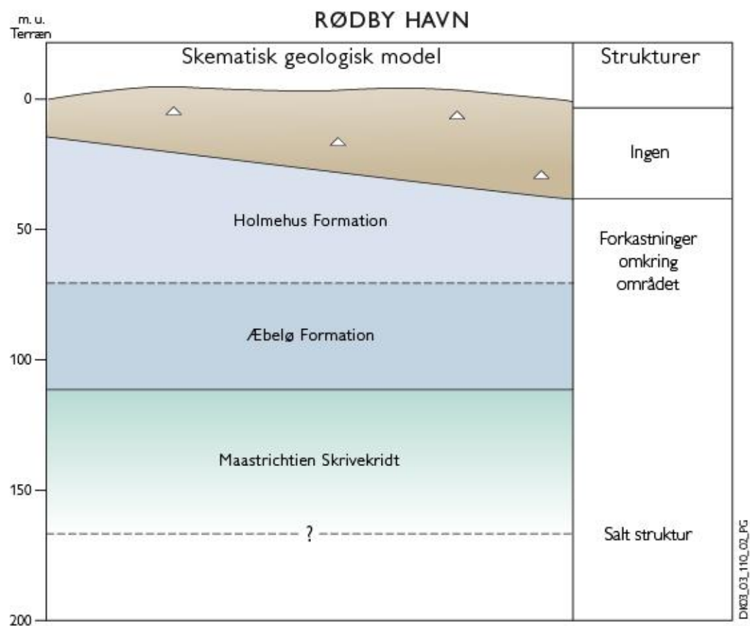
Figur 10. Skematisk geologisk model for området.
