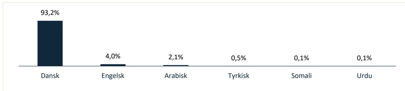
Figur 41: Sprog
